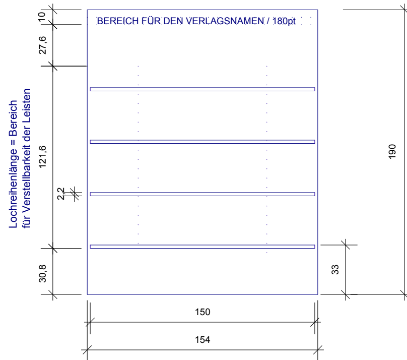
VORDERANSICHT PLATTENFLÄCHE
