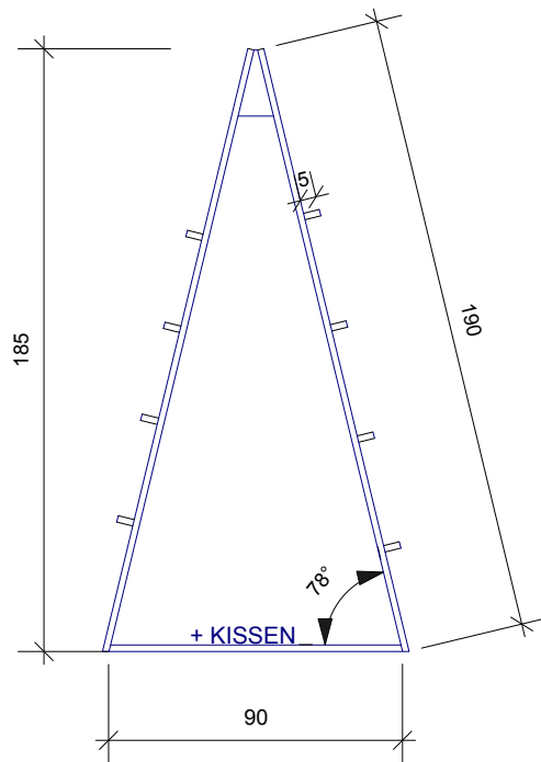
SEITENANSICHT
